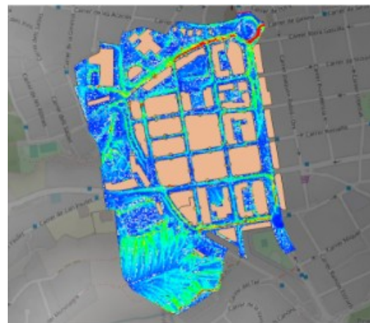
Levantamento da rede de colectores e exemplo de modelo dixital do terreo para IBER XIS e SWMM
