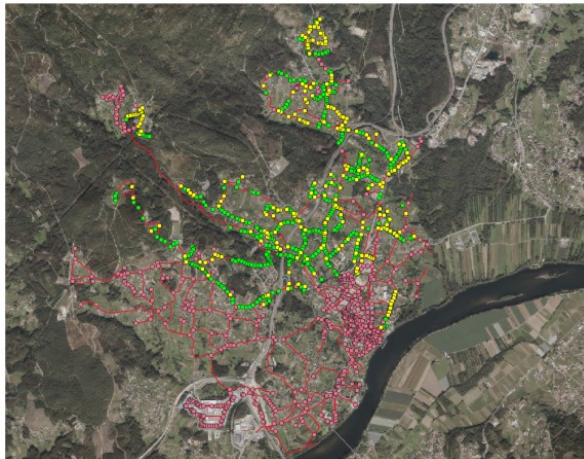
Levantamento da rede de colectores e exemplo de modelo dixital do terreo para IBER XIS e SWMM
